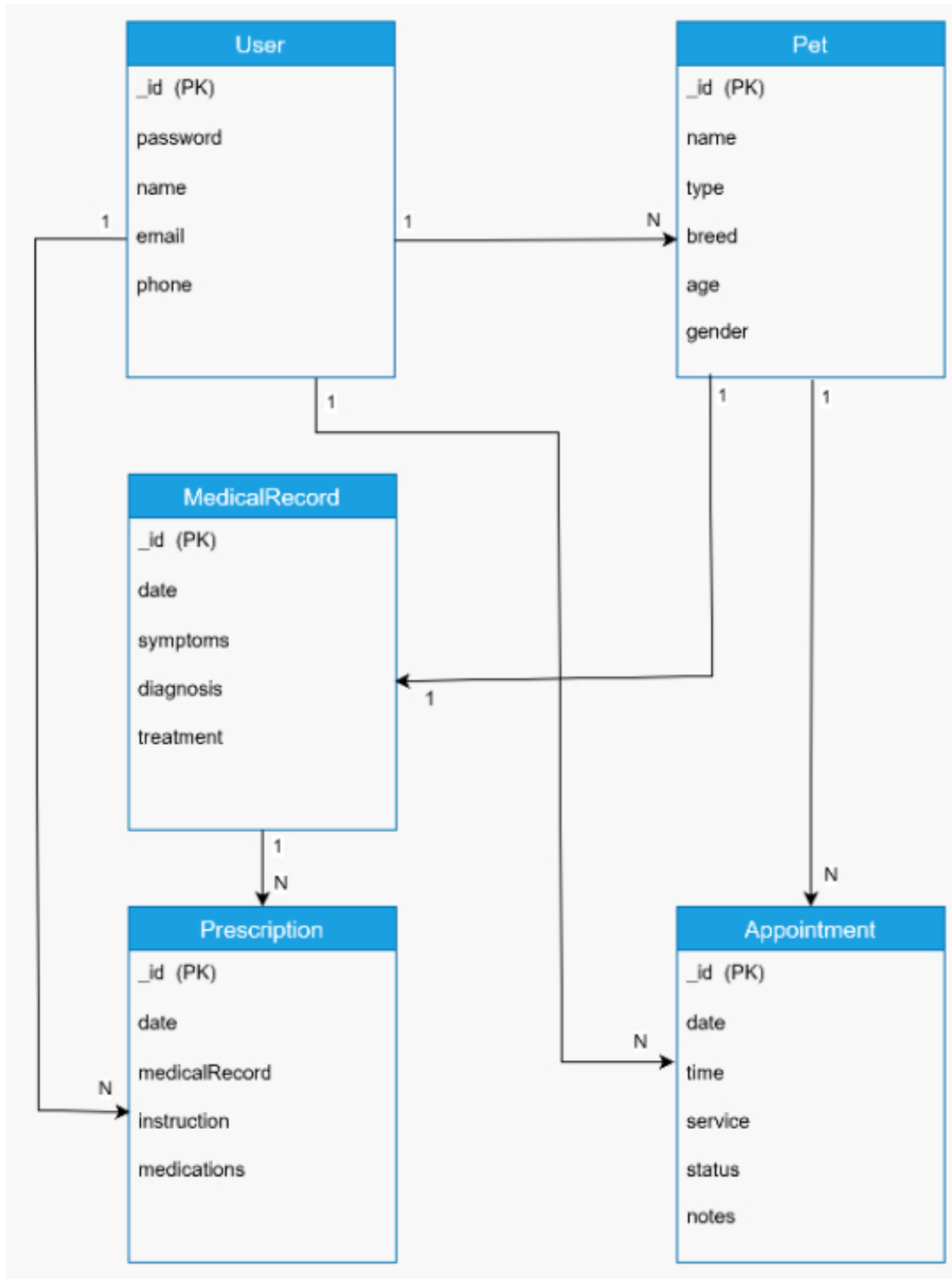
Hình 2. Logical data model (Database)
