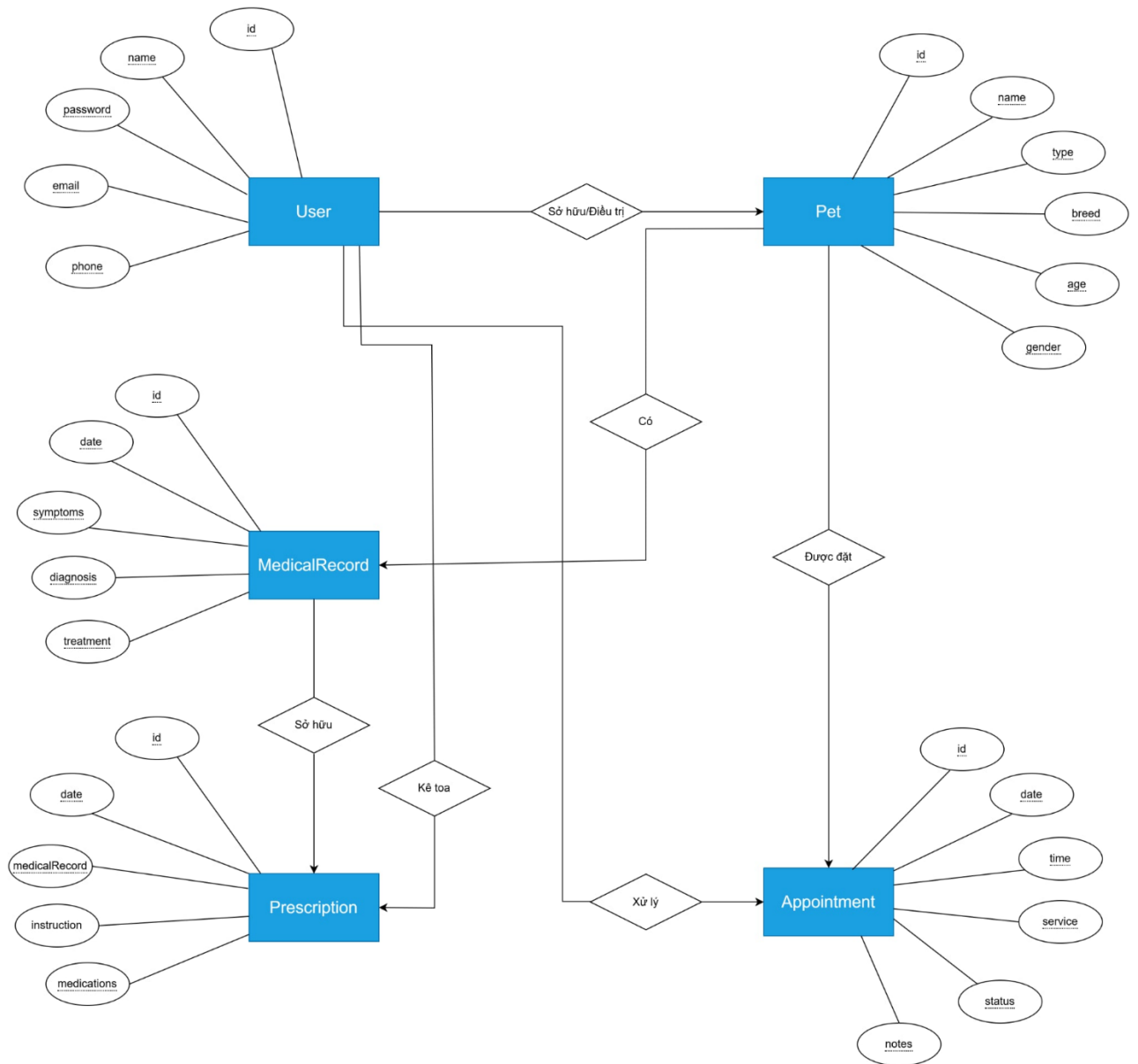
Hình 1. Sơ đồ ERD
